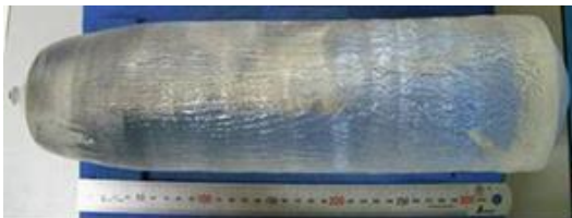
LGSO ( Lu_xGd_{(2-x)}SiO_5 )
